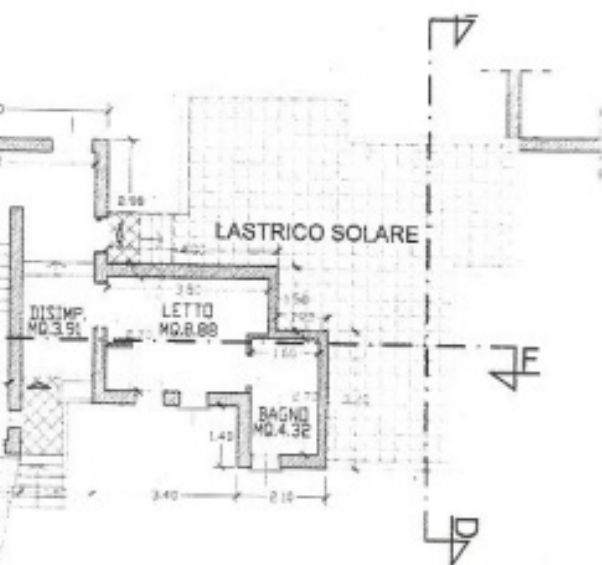
PIANTA PIANO RIALZATO STATO ATTUALE SCALA 1:100
